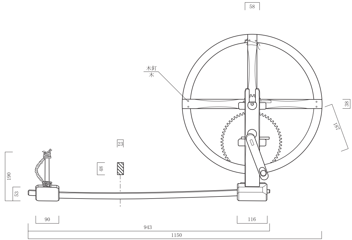
歯車説明図
