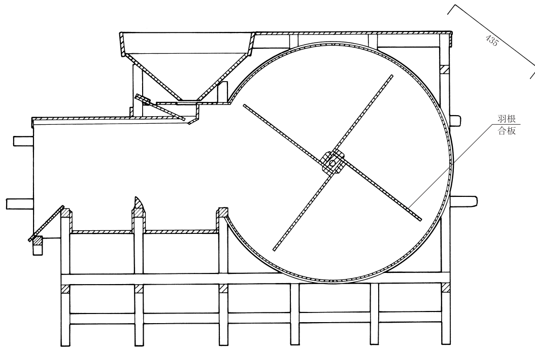
A-A' 断面図
