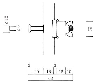
C部拡大図 (S=1/2)
