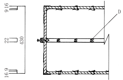
B-B' 断面図
