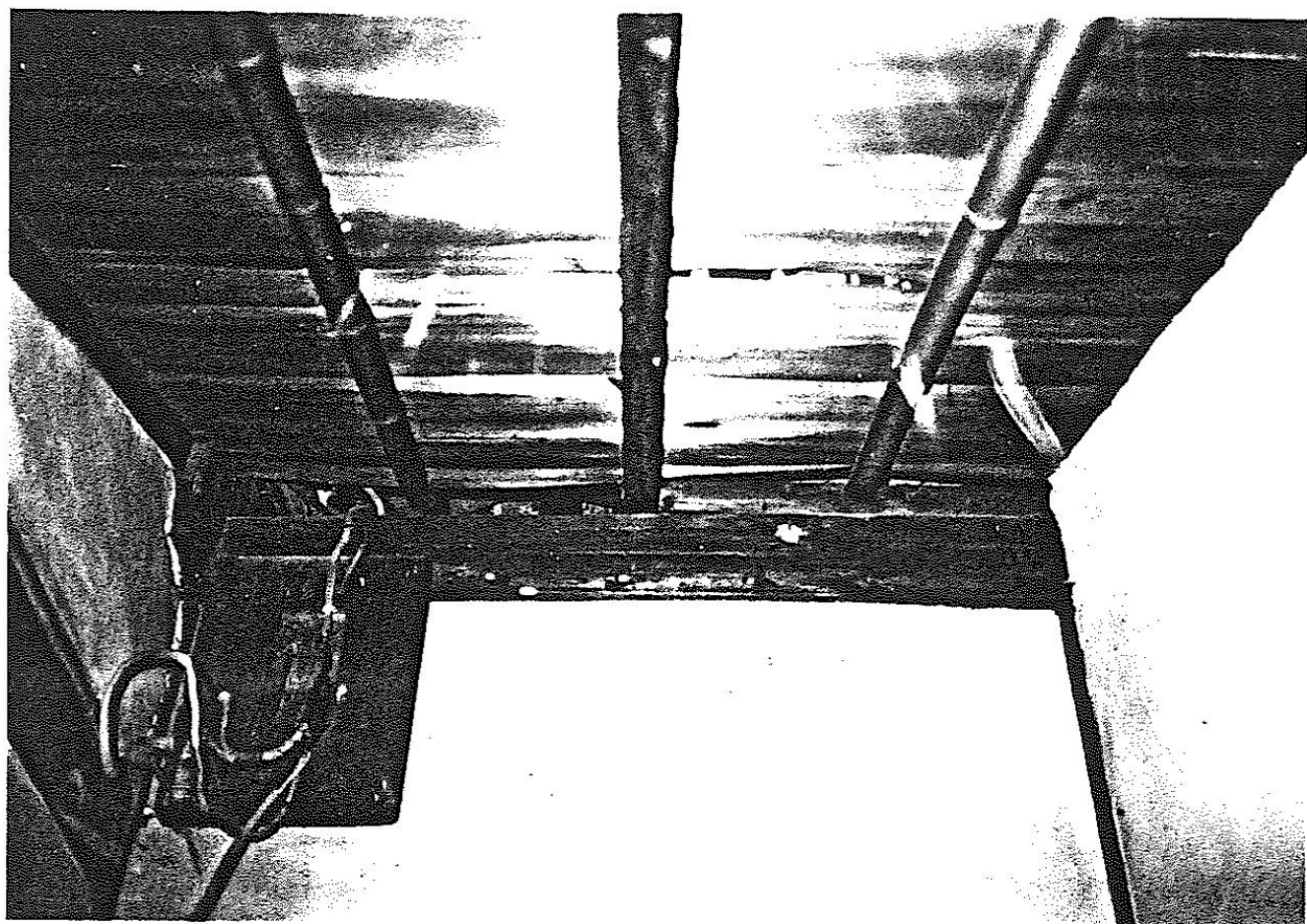
松風庵 天井と壁の 接合部分の 破損
