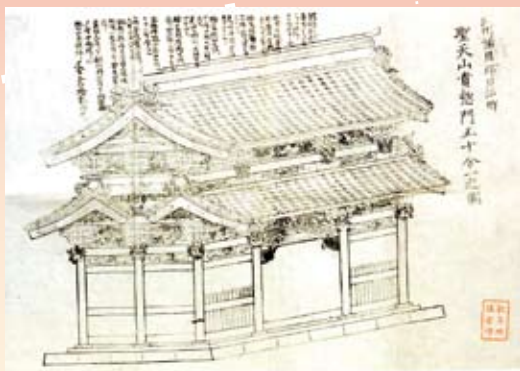
「聖天山貴惣門五十分之一図」
